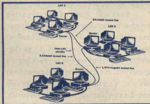
รูป แสดงการเชื่อมด้วย RO ROUTER
