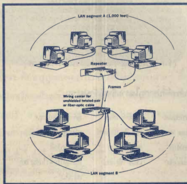
รูป แสดงการเชื่อมต่อใช้ REPEATER
