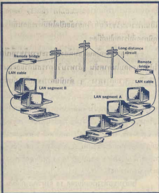
รูป REMOTE BRIDGE ของ LAN
